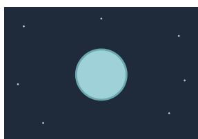
Uranus
