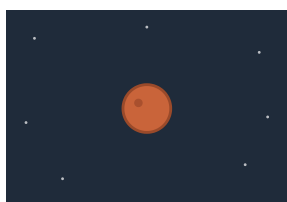
Mars
