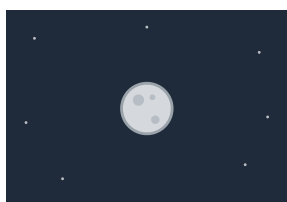
la Lune
