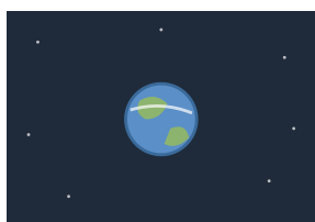
la Terre
