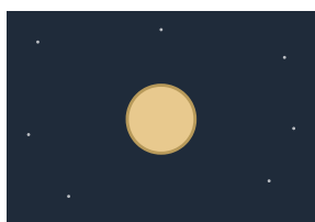
Vénus
